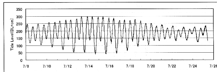
図5. 水面変位時系列 (左:観測値 右:計算値)
