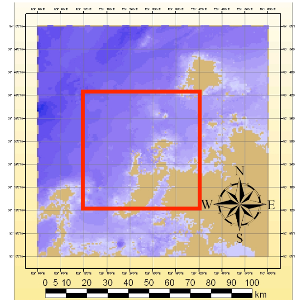
図3. 計算対象海域 (赤四角内)
